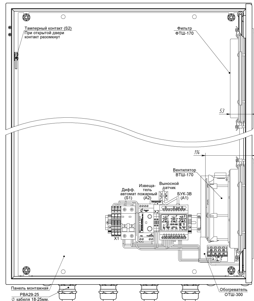
Рис.1 Устройство термощкафу (дверь открыта на 90°)
