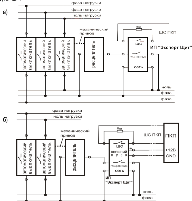
Схемы подключения ИП101/435-3-Р-Р «Эксперт Щит»
