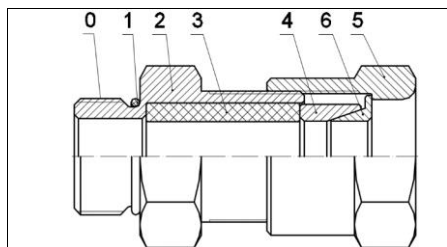
КВБ – для монтажа бронированного кабеля
