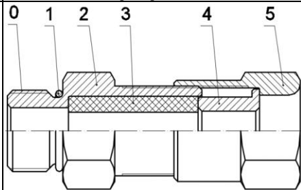
КВН – для монтажа открытого кабеля
