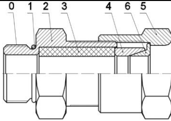
КВВ – для монтажа бронированного кабеля
