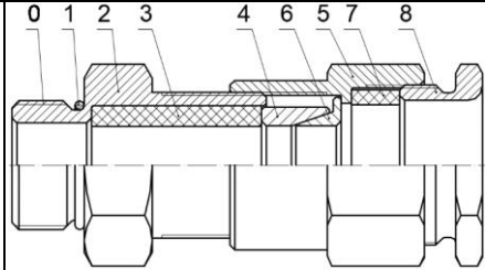
КВВ-2У – с двойным уплотнением для монтажа бронированного кабеля
