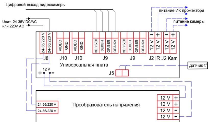
Рисунок 2 – Схема внешних подключения видеокамеры.
