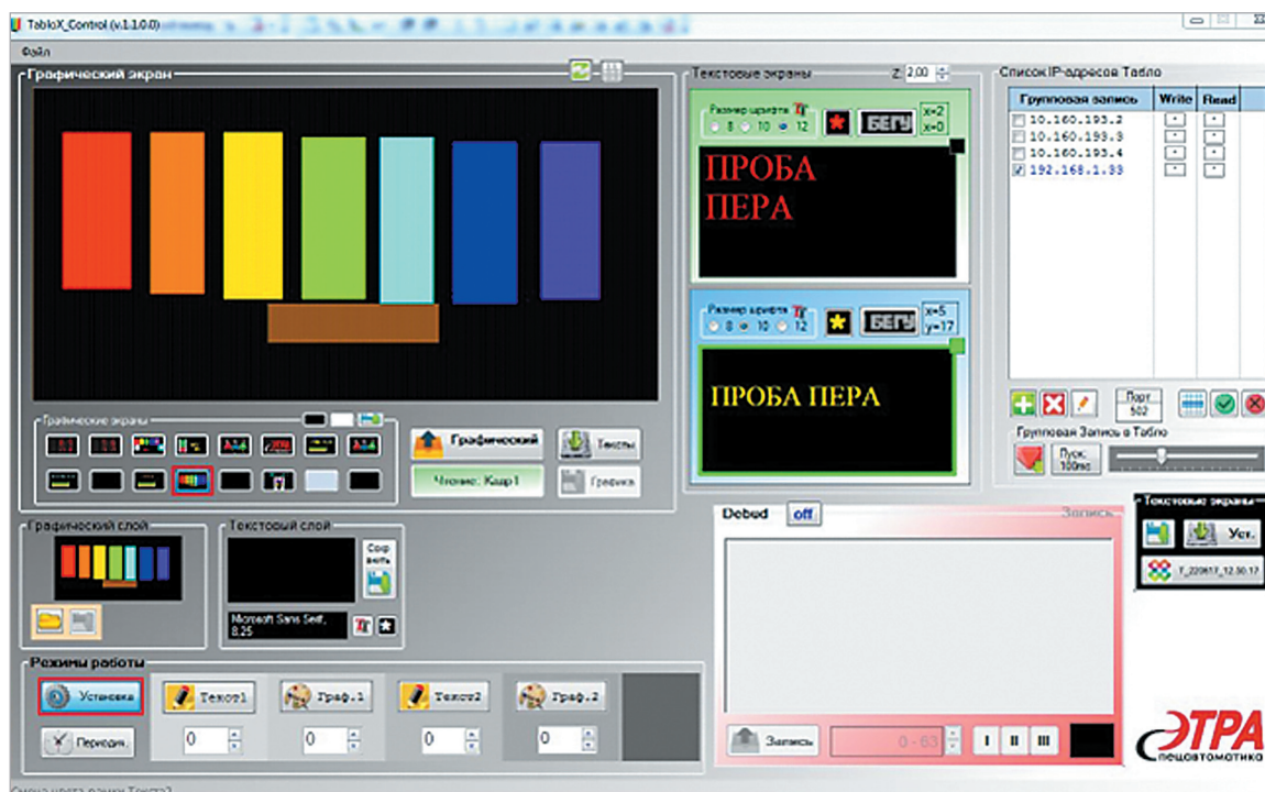
Рисунок 7. Программа TabloX_Control.
